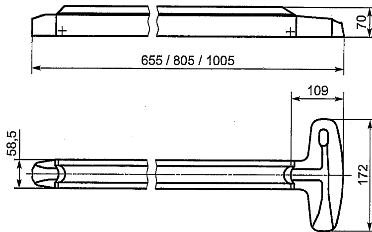
Рисунок А.2 — Пример устройства «Антипаника», управляемого штангой-рейкой для дверей эвакуационных выходов
