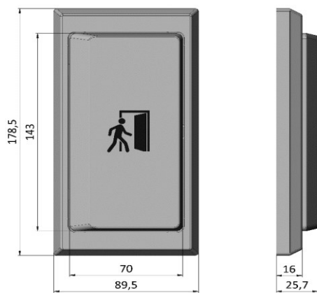
Рис. 1. Габаритные размеры
